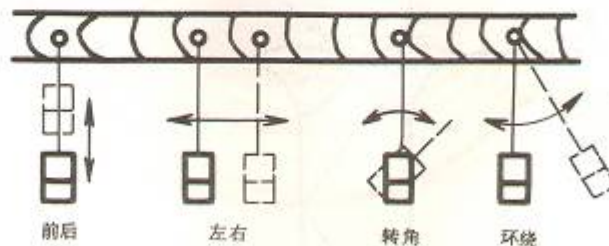
图 14 四种基本扫查方法
