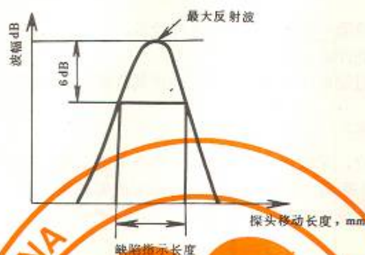
图 21 相对灵敏度测长法
