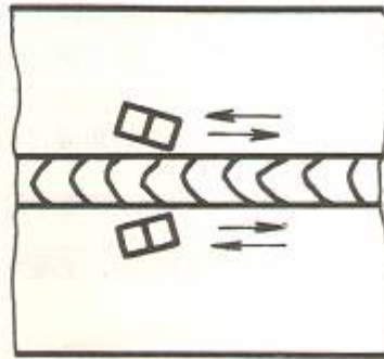
图 12 斜平行扫查
