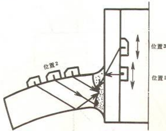
图 18 管座角焊缝
