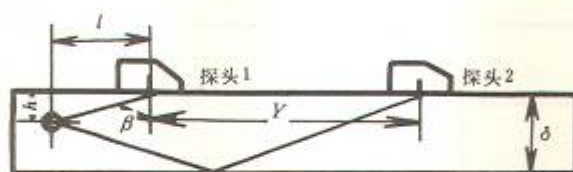
图 C3 串列扫查缺陷定位
