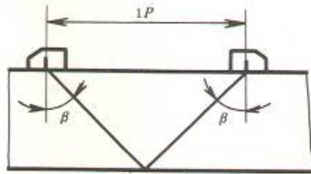
图 C1 灵敏度调节
