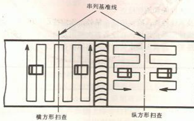
图 3 参考线
