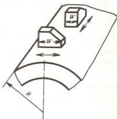
图 1 探头接触面宽度
