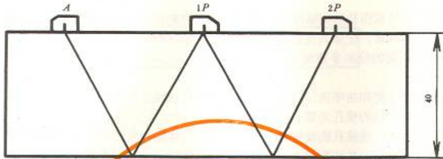
图 E 1 超声衰减的测定
