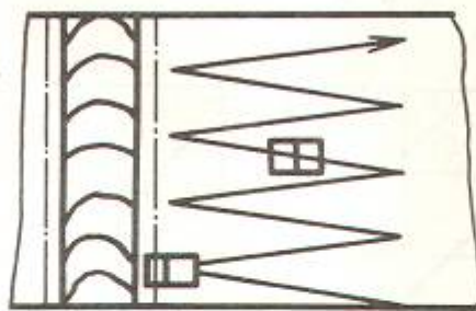
图 11 锯齿形扫查
