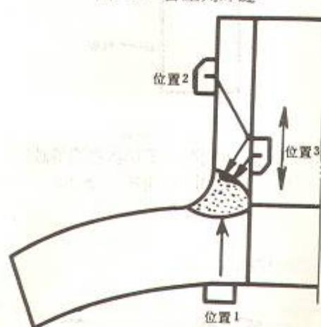
图 19 管座角焊缝
