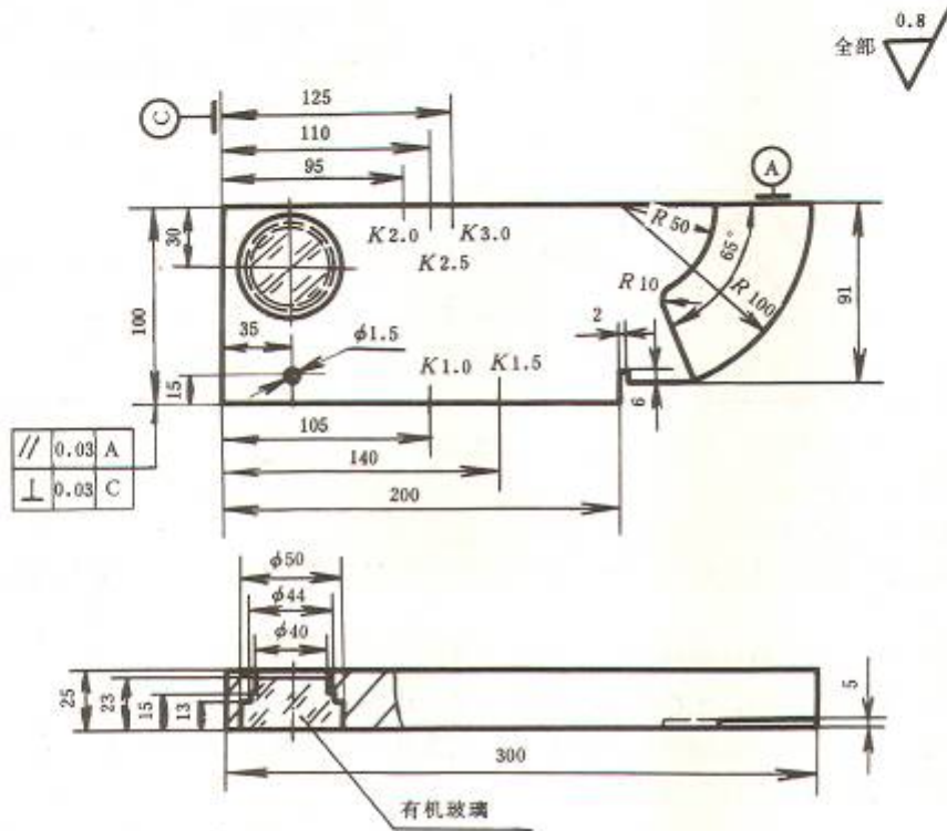
图 A1 CSK-ZB 试块
