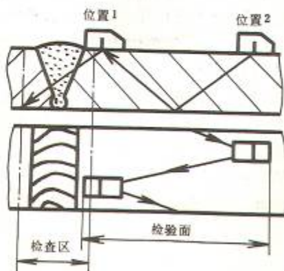
图6 检验区域
